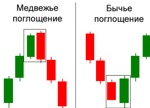
Рис. 4. Графические фигуры медвежье и бычье поглощение
