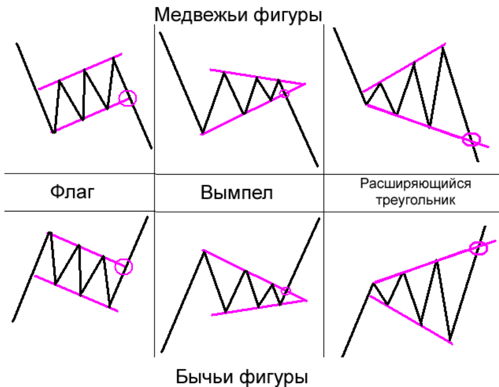
Рис. 3. Графические фигуры «флаг», «вымпел» и «расширяющийся треугольник»
