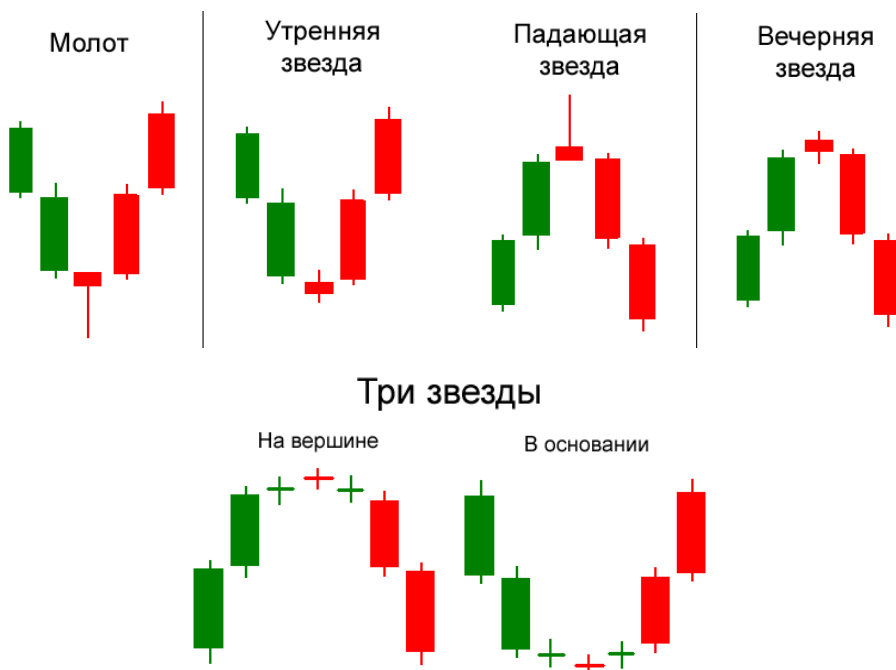
Рис. 5. Графические фигуры «три звезды», «утренняя звезда», «вечерняя звезда», «падающая звезда» и «молот»
